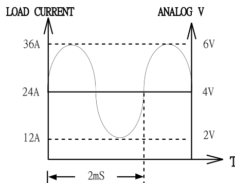
圖 2-11 負載電流之類比設定輸入
