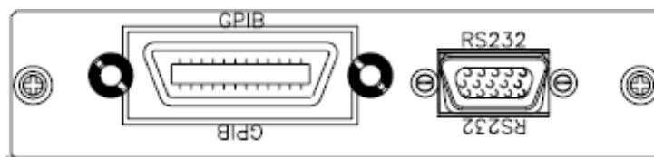
圖 2-3 3305F GPIB & RS232 連接埠圖
