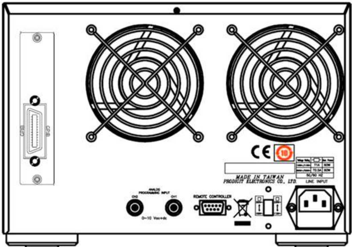
圖 3-3 3305F 後面版圖
