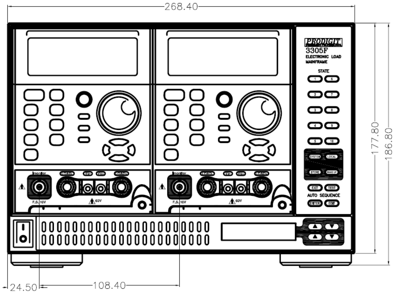
圖 3-1 3305F 前面板圖
